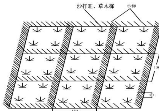
图 5-5 边坡草方格示意图（单位：cm）
