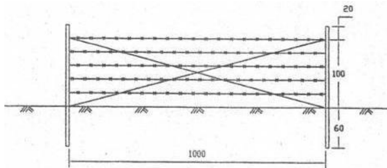
图 5-1 网围栏结构设计示意
