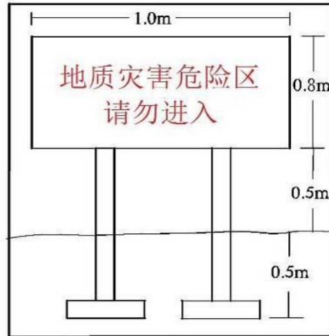
图 5-2 警示牌示意图
