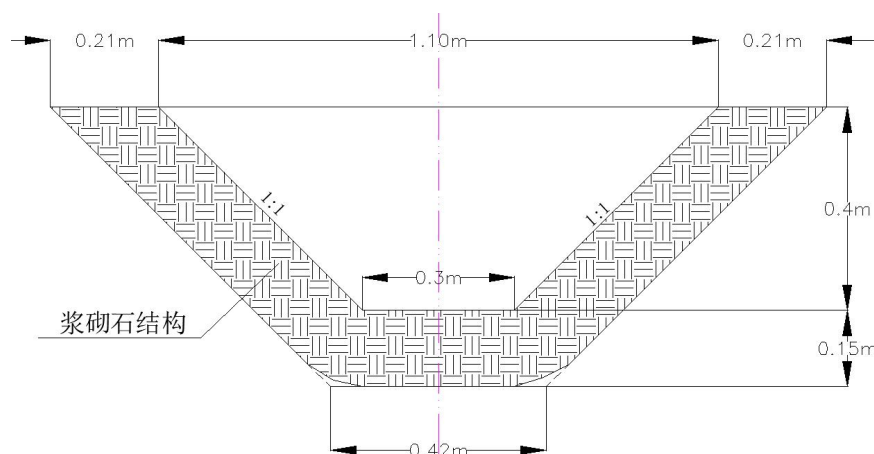
图 5-4 排水沟设计示意图（单位：cm）
