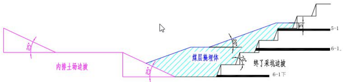
图 5-3 最终露天采坑回填掩埋煤层露头图
