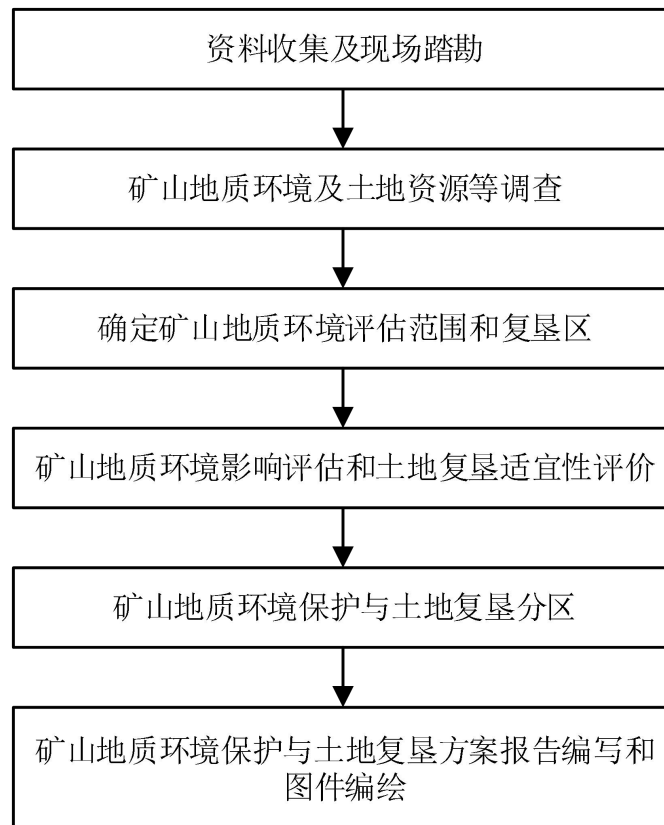
图*-* 工作程序图
